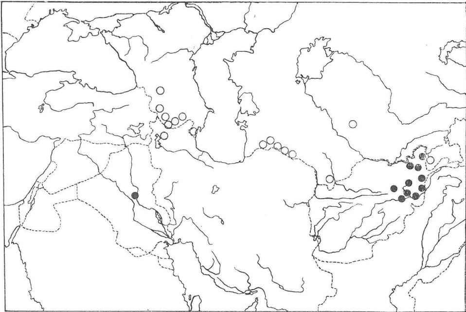
Karte 1. Verbreitung von Sphaerophoria turkmenica Bańk. ○ — Fundorte nach Literaturangaben ● — Neue Fundorte
